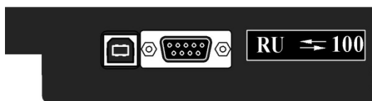
Рисунок 3 – Расположение разъемов интерфейсов USB и RS-232 на задней панели весов МК_ТН21(RU), МК_ТВ21(RU)
